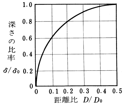
(A) 任意の点における第1フレネルゾーンの深さ
