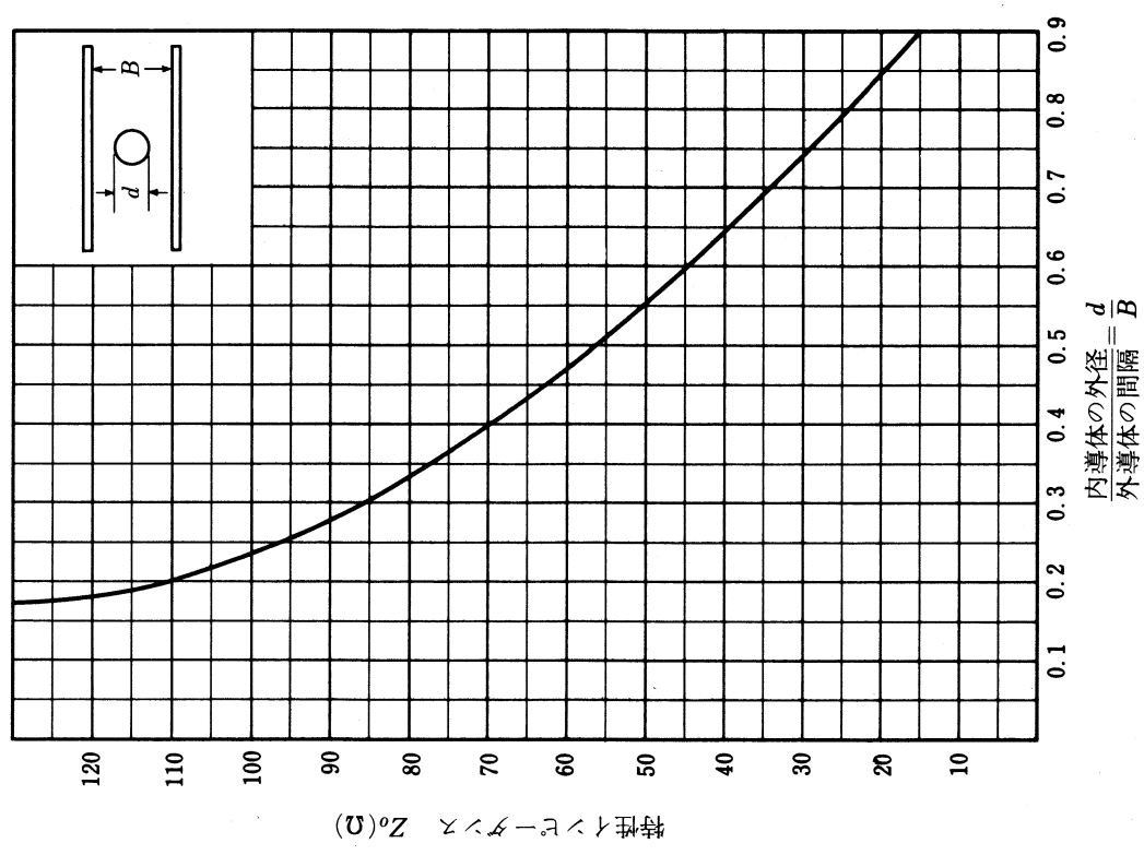
(3) 平行外導体中に内形導体を配置した線路
